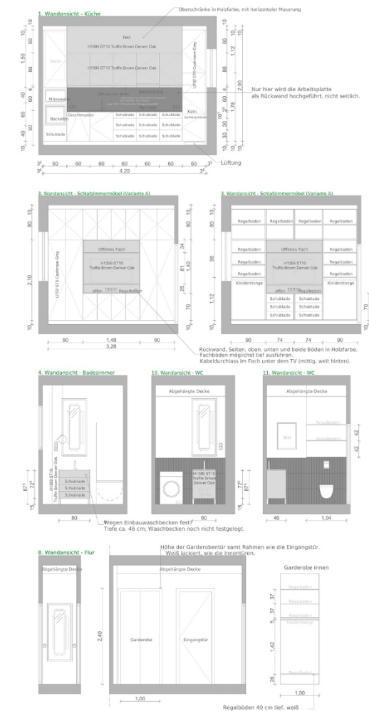
Möbelplanung-Wandansichten
