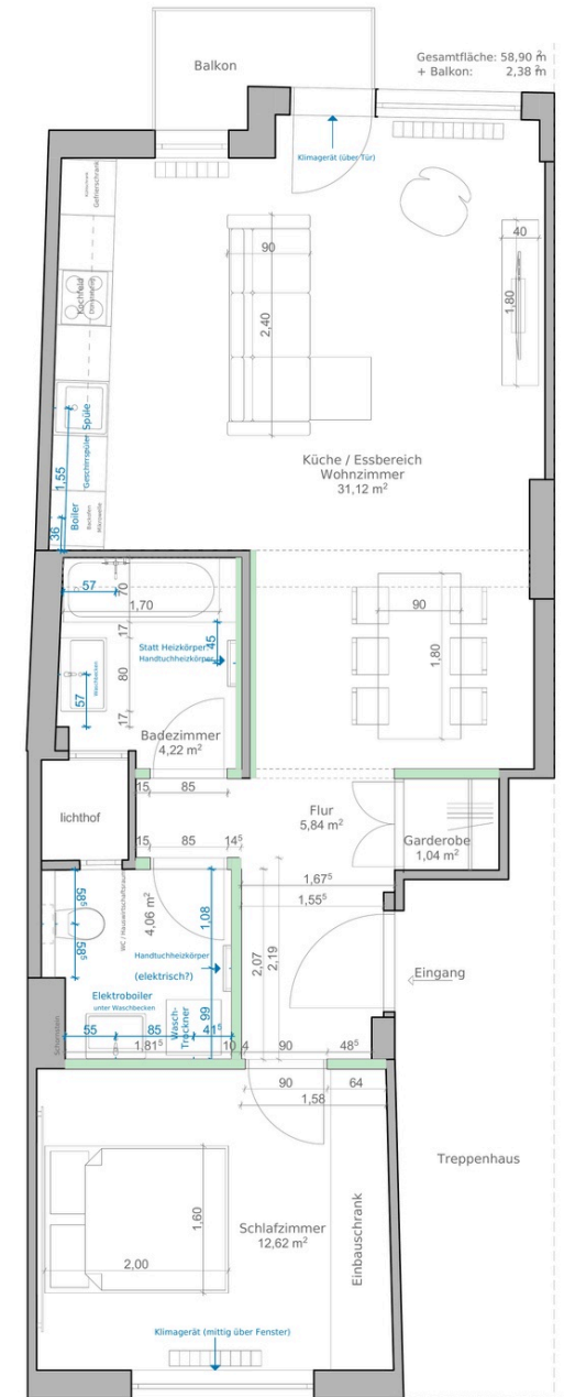
Entwurfsgrundriss
