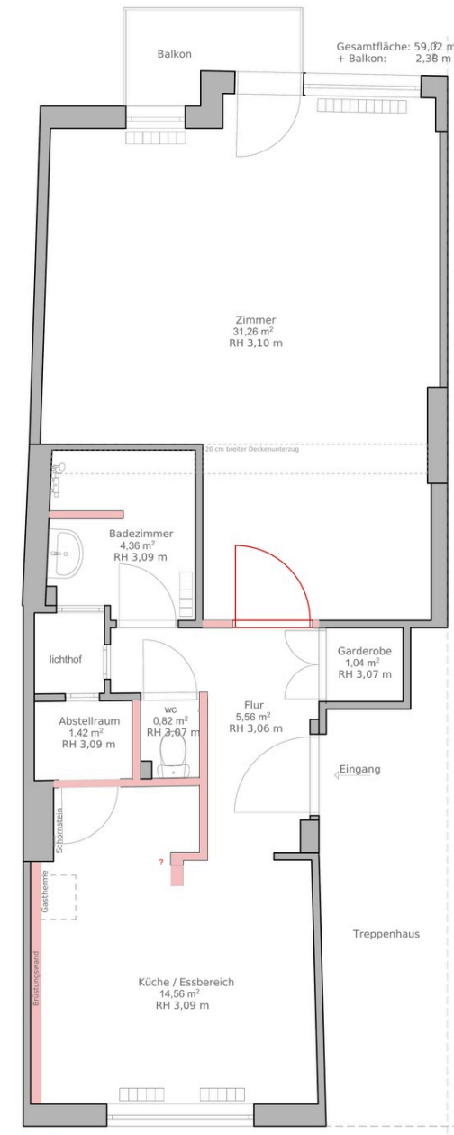
Abbruchplan
