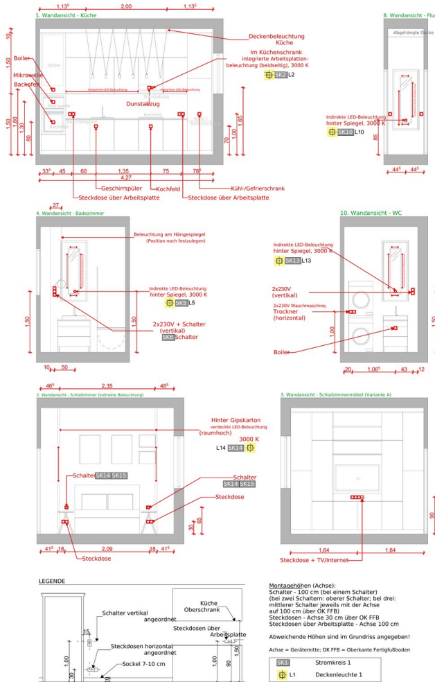
Beleuchtungsplan Wandansichten
