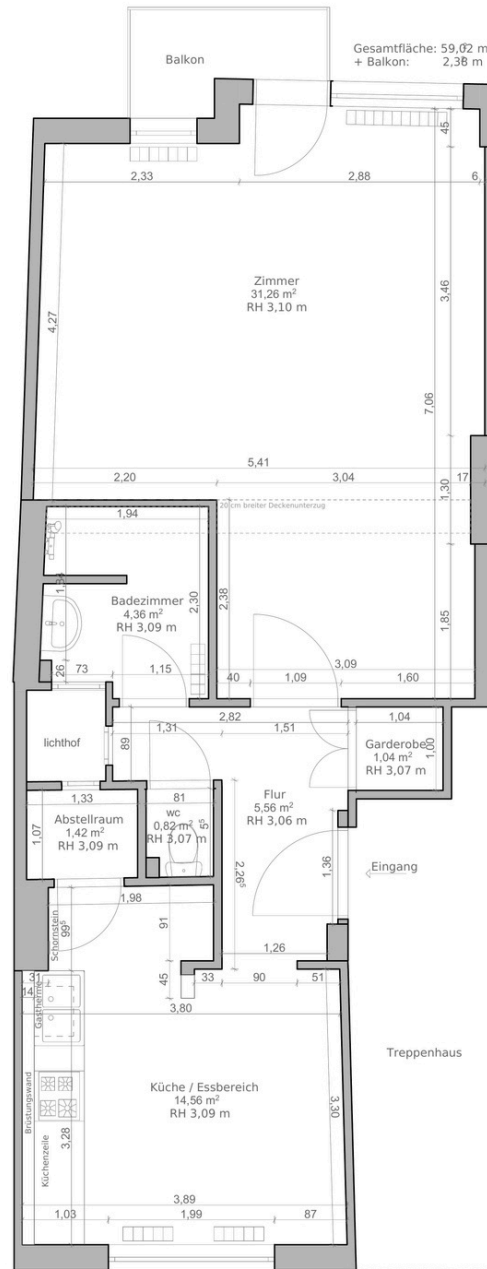
Bestandsplan
