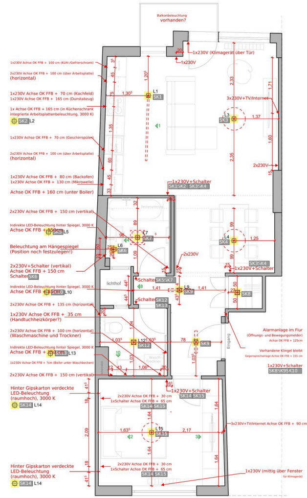
Beleuchtungsplan Grundrisse
